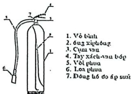
Bình bột chữa cháy MFZ
