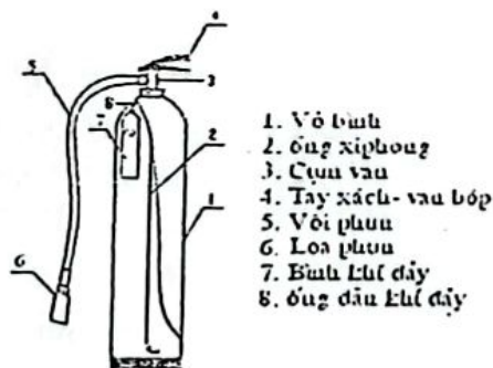
Bình bột chữa cháy MFZ
